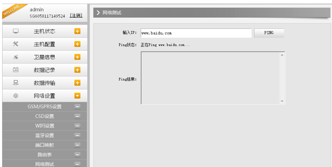
图 2.4-29 Web UI 网络设置-路由测试
